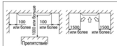
Пространство для установки и обслуживания
