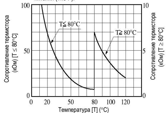
Температурная характеристика сопротивления термистора транзистора питания (Tho-P).
