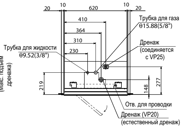
Пространство для установки и обслуживания
